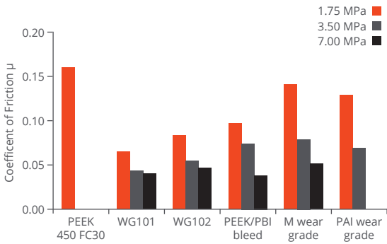
图11: 各种F10PEEK材料与其他高性能材料相比的在1m / s测试速度下使用止推垫圈方法测试的摩擦系数
