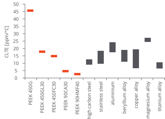
图8:各种F10PEEK材料相对于金属的线性热膨胀系数(CLTE) (流动方向, 低于Tg)
